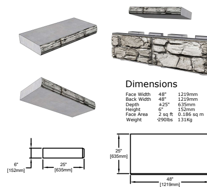
CAP UNIT
